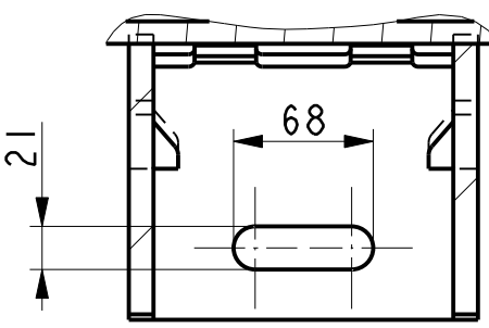
COUPE PARTIELLE B-B PARTIAL SECTION B-B
